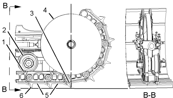
Рисунок 3 g02589156 Для большей наглядности часть узлов и деталей не показана. При измерении размера (A) необходимо соблюсти следующие условия. Рельсовые направляющие (1) должны контактировать со всеми катками (2) по всей длине машины. Для измерения высоты подъема (A) грунтозацепа (3) необходимо, чтобы он находился непосредственно под центром переднего направляющего колеса (4). Участок гусеничной ленты (5) между передним направляющим колесом и передним нижним катком должен быть ровным и горизонтальным. Грунтозацепы (6) под нижними катками должны лежать на ровной горизонтальной поверхности.
